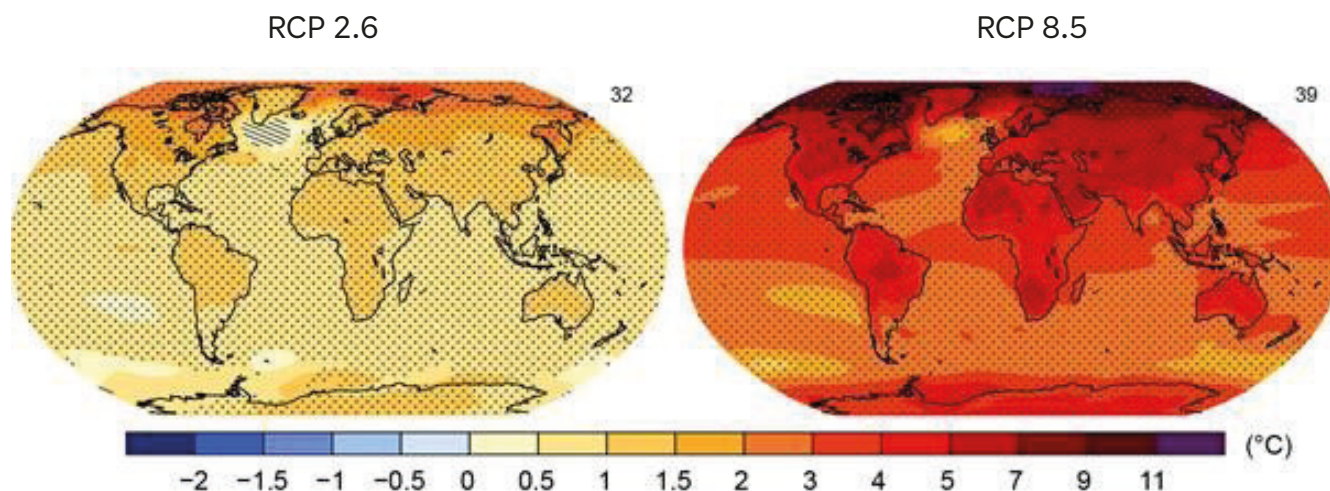
Figur 1: Globale temperaturendringer. Endringer i gjennomsnittlig overflatetemperatur på jorda fra 1986-2005 til 2081-2100. Kilde: FNs klimapanel 2013/Miljøstatus.no
