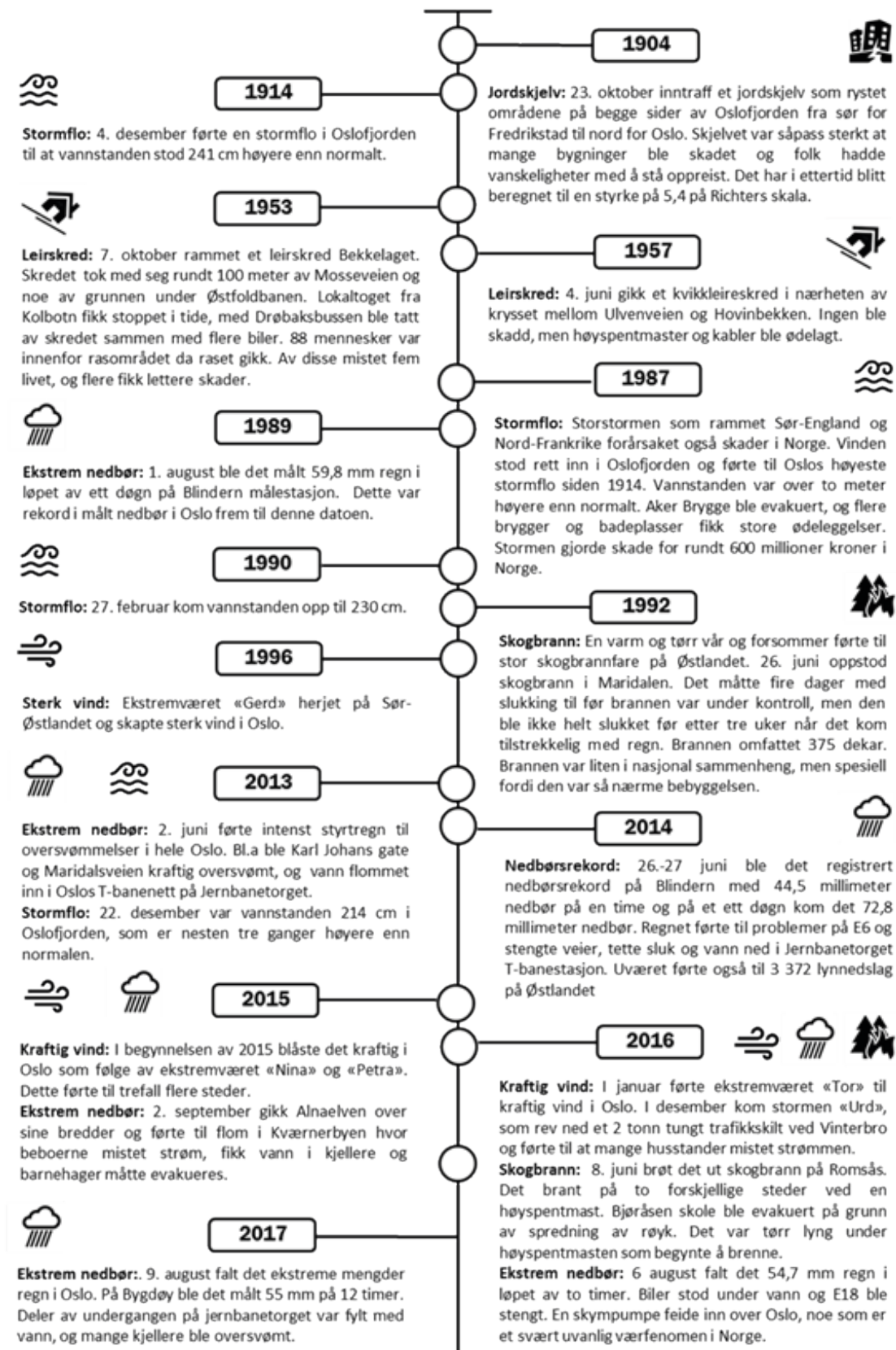
Figur 3:: Utvalgte ekstreme naturhendelser i Oslo fra 1900 til i dag.
