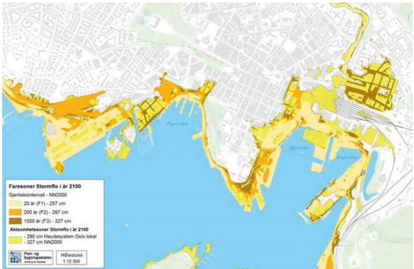
Figur 5: Utdrag av faresonekart for stormflo i 2100 (Plan- og bygningssetaten i Oslo)
